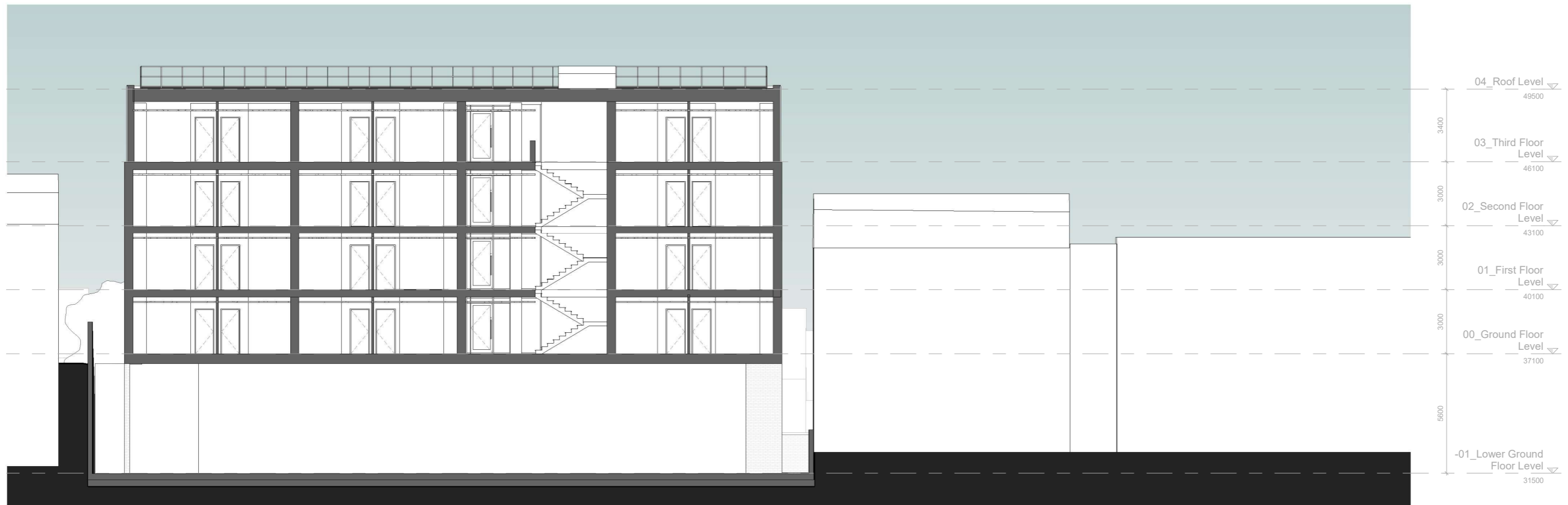
Section AA 1 : 100
